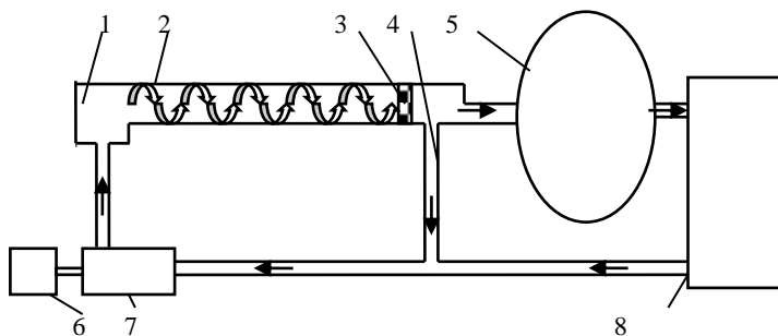
Рис. 1 Схема теплогенератора, работающего на принципе закрутки воды: 1- улитка; 2- труба цилиндрическая; 3- турбулизатор; 4- байпасная линия; 5- промежуточная емкость; 6- электродвигатель; 7- насос; 8- тепло radiаторы.
